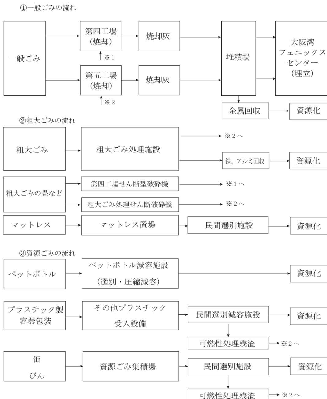
図1-7 搬入ごみの処理の流れ
