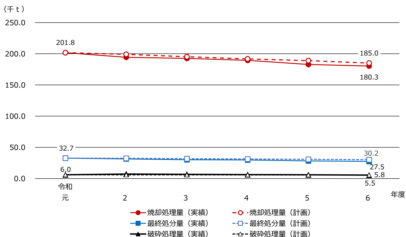
図1-27 焼却処理量・破碎処理量・最終処分量の計画値と実績値の比較
