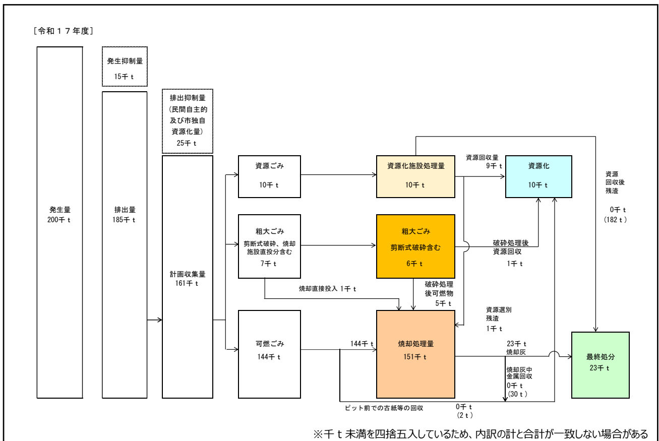
図3-6 ごみ処理の流れ（令和6年度・令和17年度）
