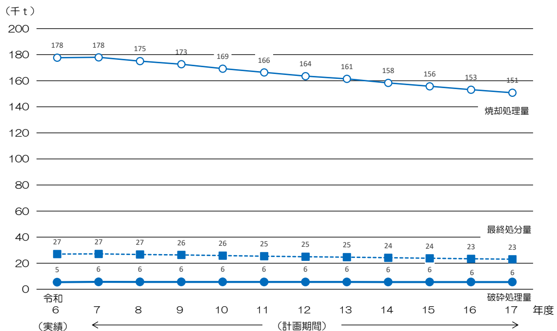
図3-5 焼却処理量・破碎処理量・最終処分量の推移予測
