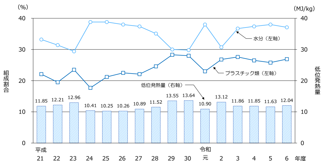
図1-16 搬入ごみ質の変化
